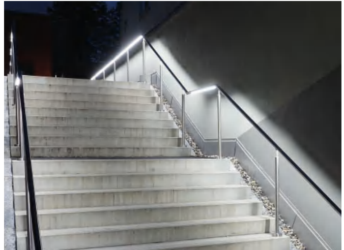
LaneLED INOX42, Lindenplatz square Baden
